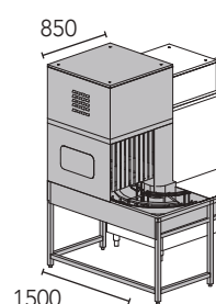
KDRA184MT 4,5 kW électrique KDRA189MT 9 kW électrique Séchage sur virage motorisé 180°
