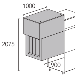
KDR94 4,5 kW électrique KDR99 9 kW Electrique Séchage
