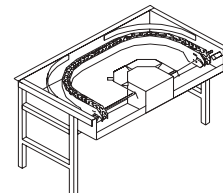
K23 850x1500x885 H Virage motorisé 180° ( horaire et antihoraire )
