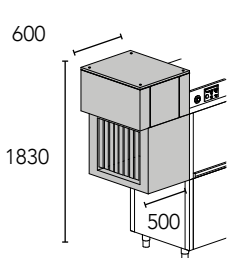
KDR24 4,5 kW Asciugatura
